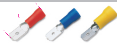
1620R/6,3K 0,5+1,5 mm 2 HxS 6,3x0,8 mm
